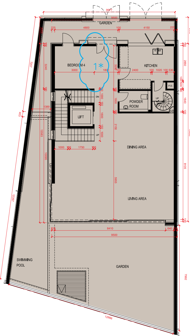
Ground Floor Plan 地下平面圖
