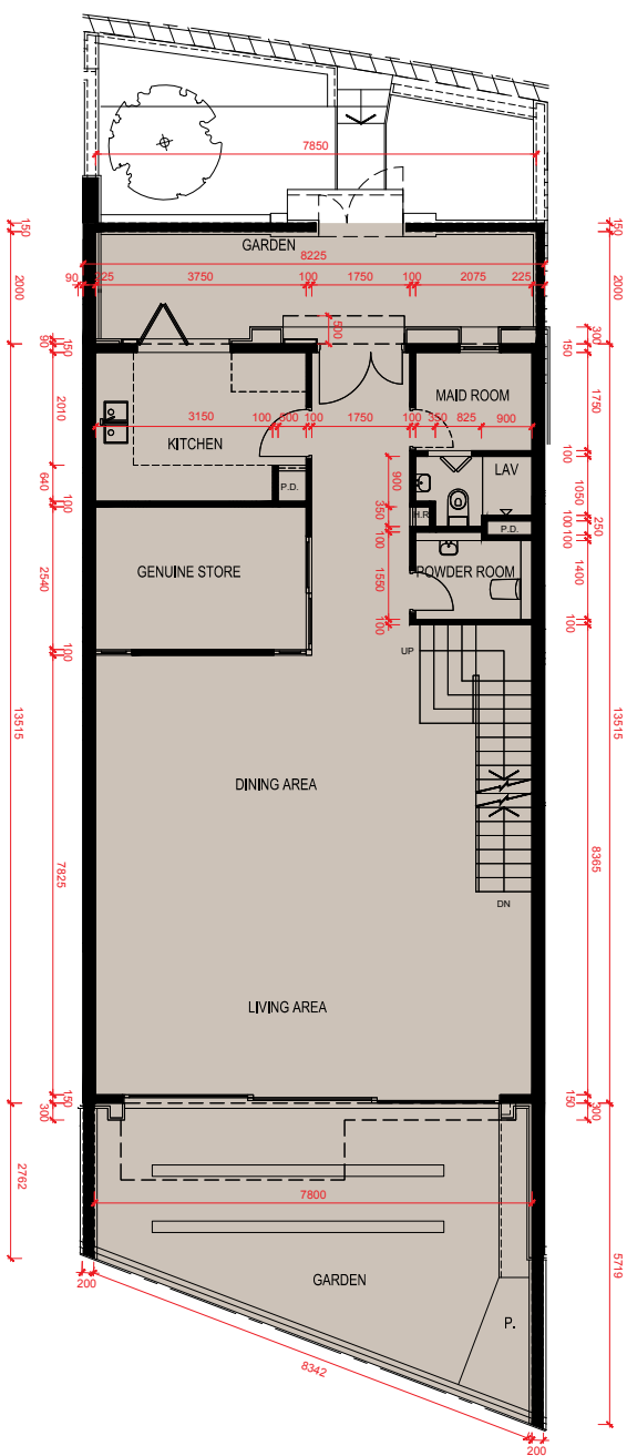
Ground Floor Plan 地下平面圖
