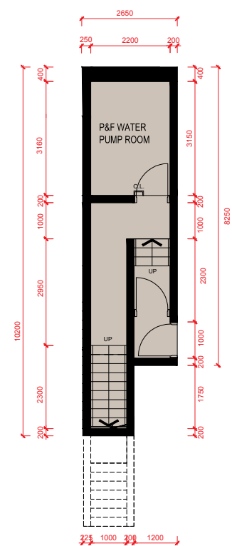
Carpark Floor Plan 停車場平面圖
